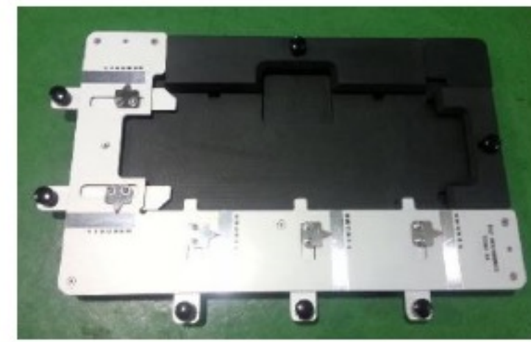
중대형 전지 측정,검사 지그
